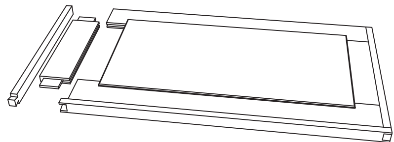
Lid explode
